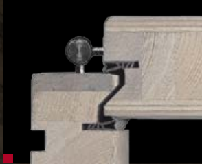
WRĘG ANTYWYWAŻENIOWY
