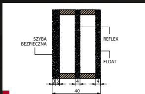
ZESTAW SZYBOWY BEZPIECZNY O GRUBOŚCI 40 mm ZE SZKŁEM „REFLEX”
