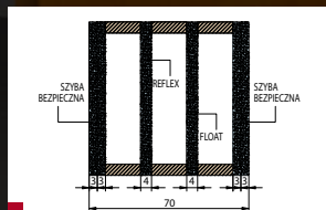
ZESTAW SZYBOWY BEZPIECZNY O GRUBOŚCI 70 mm ZE SZKŁEM „REFLEX”
