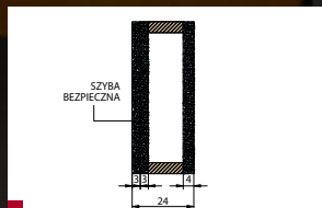
ZESTAW SZYBOWY BEZPIECZNY O GRUBOŚCI 24 mm ZE SZKŁEM „REFLEX”
