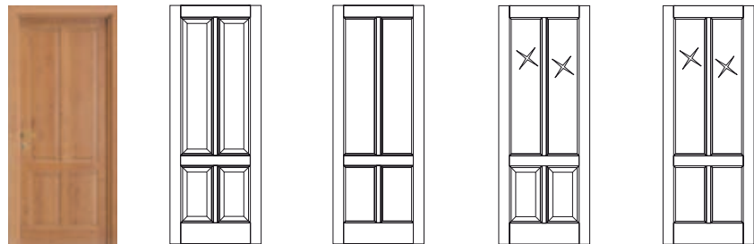
STR. 31 PEŁNE Z LITEGO DREWNA PEŁNE Z PŁYCINĄ MDF FORNIROWANĄ PRZESZKLONE Z PŁYCINĄ ANGIELSKIE Z PŁYCINĄ MDF FORNIROWANĄ
