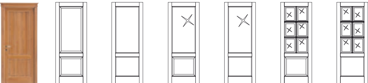
STR. 30 PEŁNE Z LITEGO DREWNA PEŁNE Z PŁYCINĄ MDF FORNIROWANĄ PRZESZKLONE Z LITEGO DREWNA PRZESZKLONE Z PŁYCINĄ MDF FORNIROWANĄ ANGIELSKIE Z LITEGO DREWNA ANGIELSKIE Z PŁYCINĄ MDF FORNIROWANĄ
