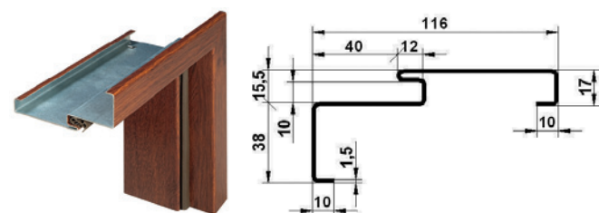
Ościeżnica FT SL, narożnikowa z uszczelką (do drzwi metalowych STANDARD WD, C, S)
