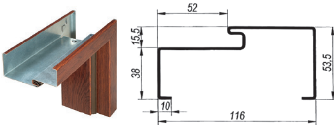
Ościeznica FA Premium SL, asymetryczna z uszczelką (do drzwi panelowych PREMIUM WX10, CX10, SX10)
