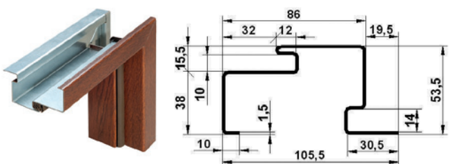
Ościeżnica FR SL, asymetryczna portalowa z uszczelką (do drzwi panelowych STANDARD WX10, CX10, SX10)
