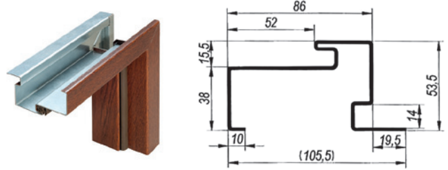
Ościeznica FR Premium, asymetryczna z uszczelką (do drzwi metalowych PREMIUM WD, C, S)
