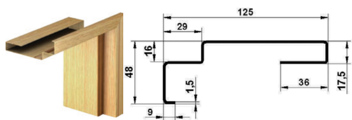
Ościeżnica FN, narożnikowa bez uszczelki (do drzwi metalowych STANDARD WD, C, S)
