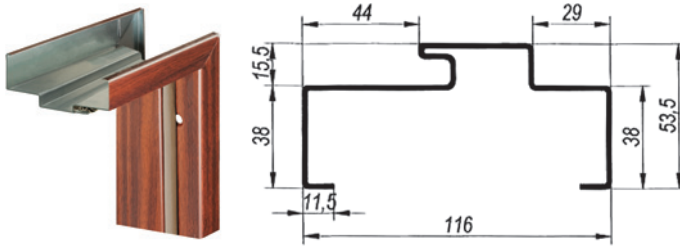
Ościeznica FC Premium z uszczelką (do drzwi metalowych PREMIUM WD, C, S)
