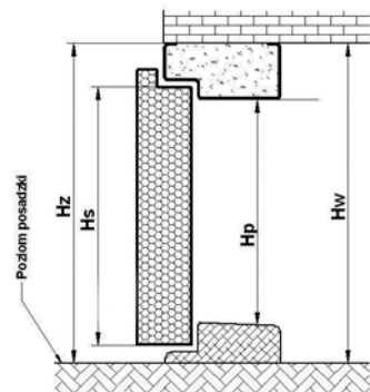
Rysunek poglądowy dla ościeżnic drzwi i progów dla: FD, FC, FC SL, FR, FR SL, FA SL
