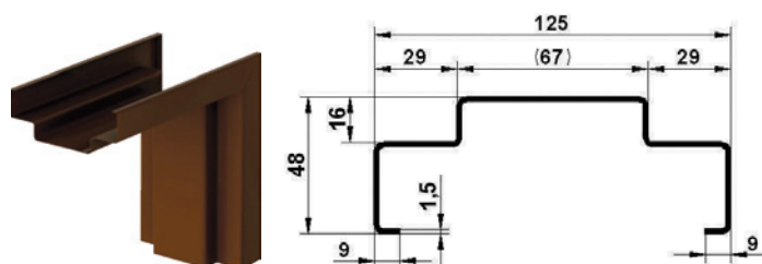
Ościeżnica FD bez uszczelki (do drzwi metalowych STANDARD WD, C, S)
