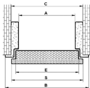
Rysunek poglądowy dla ościeżnic FN, FT SL
