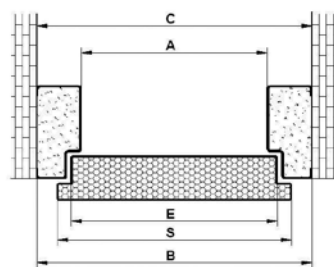
Rysunek poglądowy dla ościeżnic FC, FC SL, FD, FR, FR SL, FA SL
