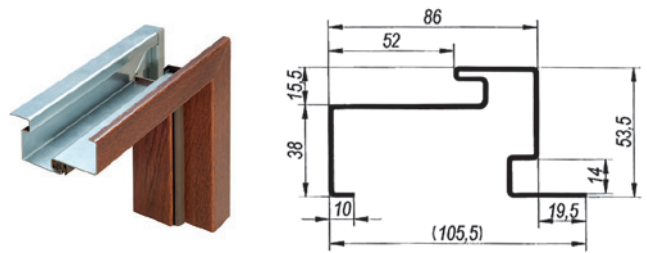
Ościeznica FR Premium SL, asymetryczna z uszczelką (do drzwi panelowych PREMIUM WX10, CX10, SX10)
