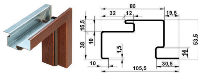
Ościeżnica FR, asymetryczna portalowa z uszczelką (do drzwi metalowe STANDARD WD, C, S)
