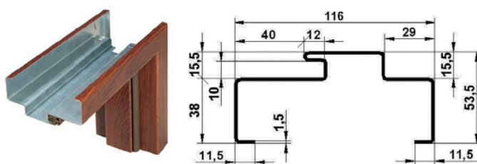
Ościeżnica FC SL z uszczelką (do drzwi panelowych STANDARD WX10, CX10, SX10)
