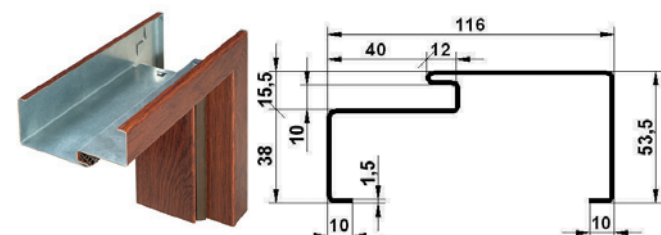
Ościeżnica FA SL, asymetryczna z uszczelką (do drzwi panelowych STANDARD WX10, CX10, SX10)
