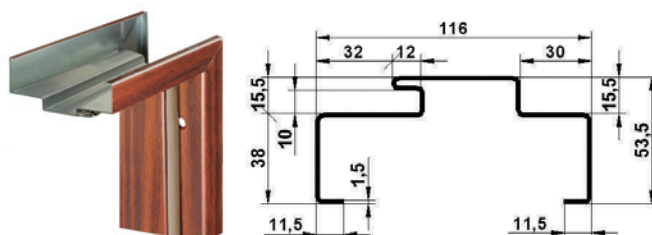
Ościeżnica FC z uszczelką (do drzwi metalowych STANDARD WD, C, S)
