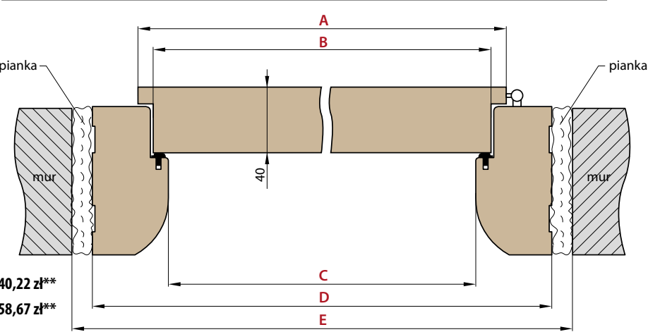
SCHEMAT OŚCIEŻNICY STAŁEJ
