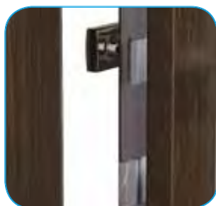
zamek listwowy czteropunktowy dostosowany pod dwie wkładki patentowe
