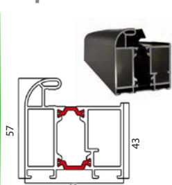
Ościeżnica TERMO
